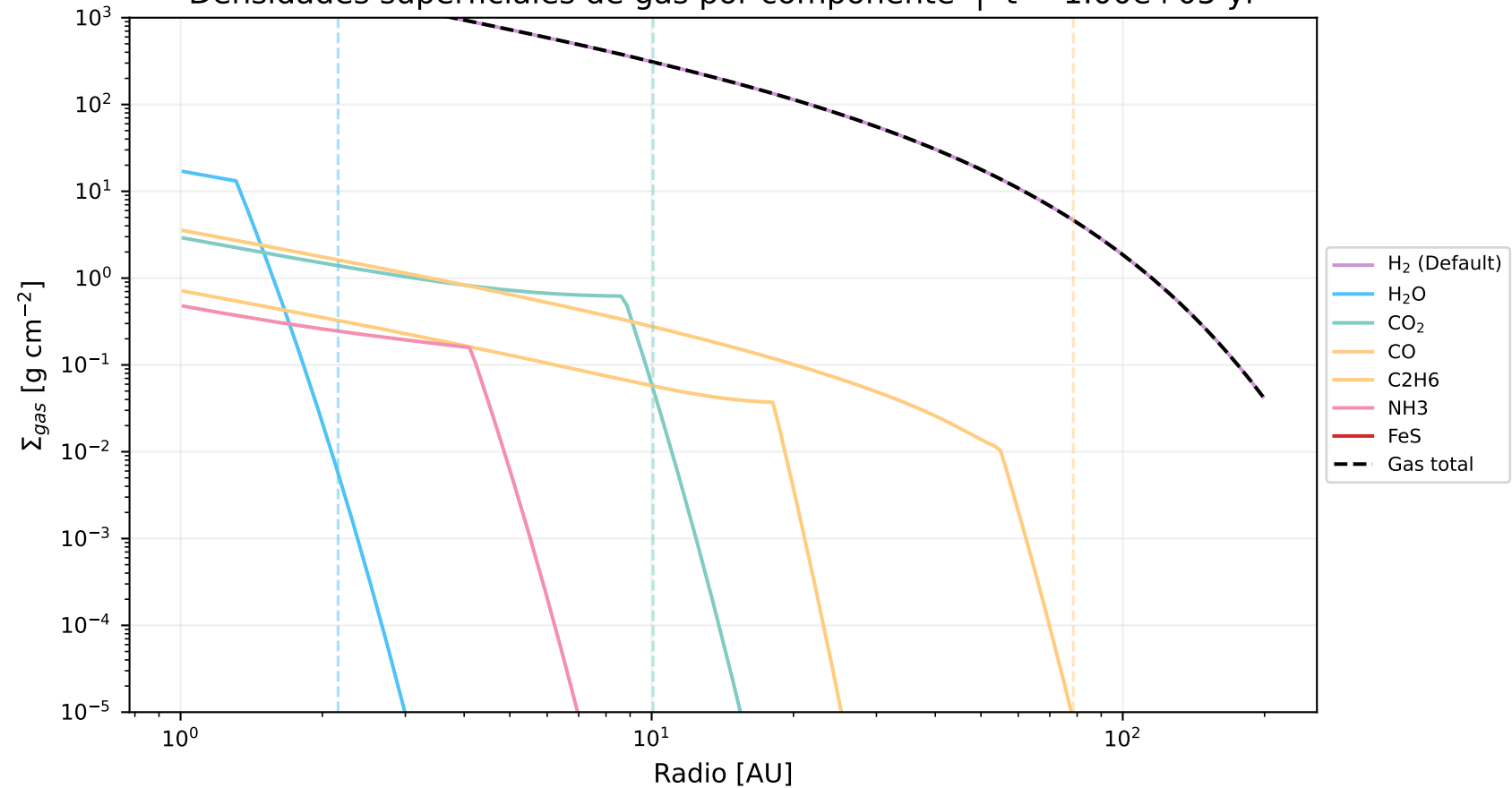
Densidades superficiales de gas por componente | t = 1.00\text{e}+05 \text{ yr}
